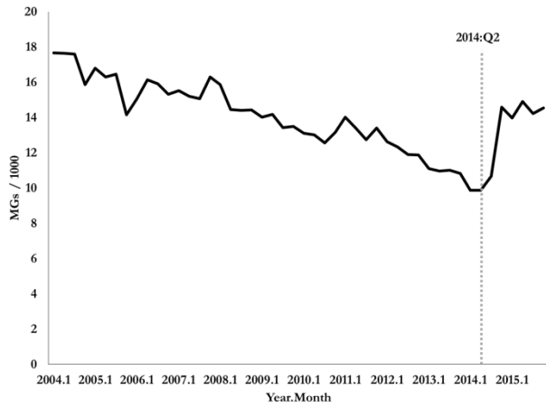
c: Codeine
