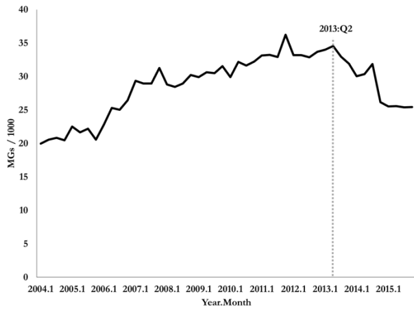
a: Hydrocodone
