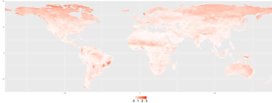
(d) RCP 8.5
